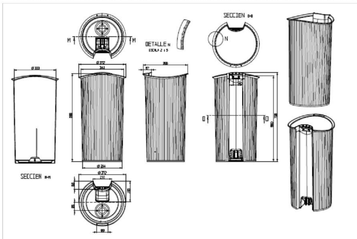
Ilustración 13. Planimetría cesta prototipo tipo A para el almacenamiento residuos generados por transeúntes.
