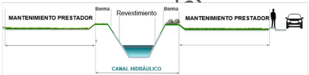
Ilustración 20. esquema de los canales de aguas lluvias.
