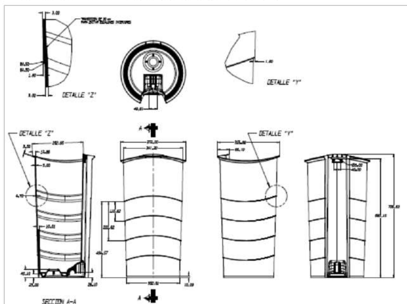
Ilustración 15. Planimetría prototipo tipo B caneca
