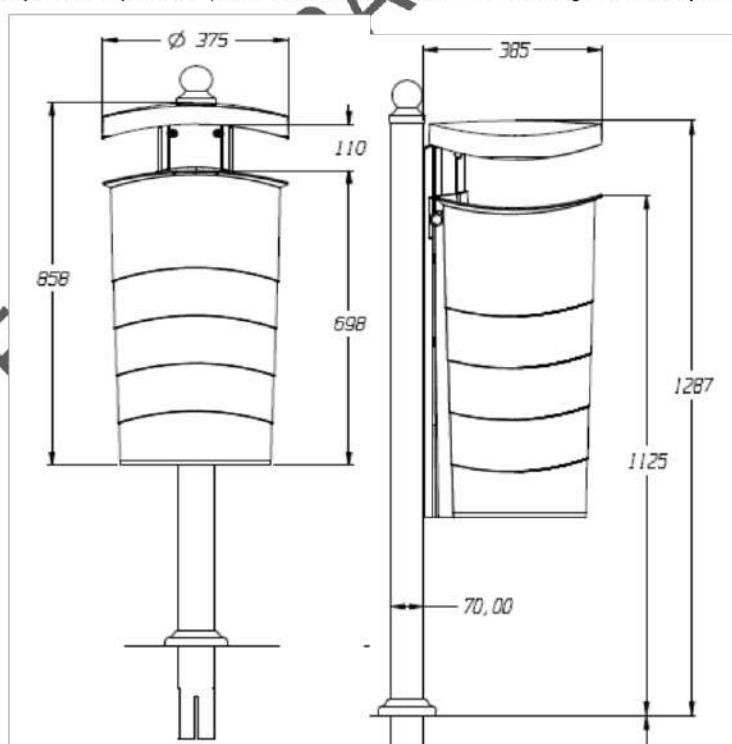
Ilustración 14. Prototipo cesta pública para el almacenamiento residuos generados por transeúntes.
